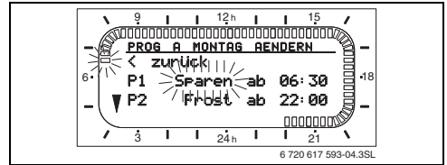
Bild 14 Betriebsart einstellen
