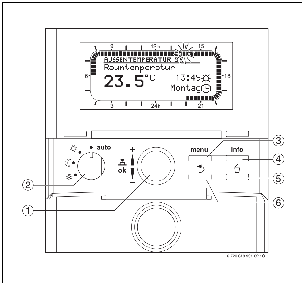
Bild 3 Bedienelemente bei geöffneter Klappe
