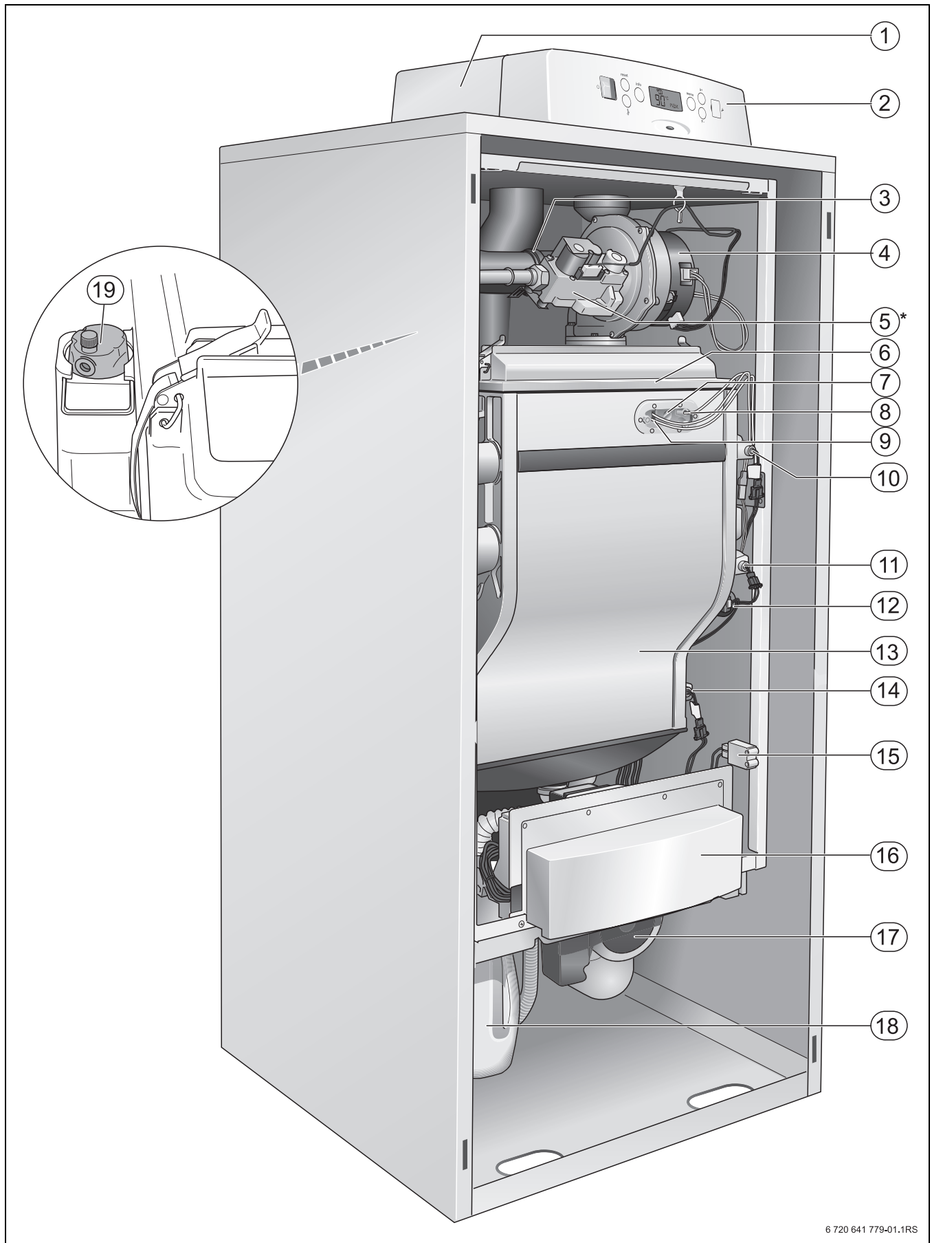
Bild 1 Produktübersicht Suprapur KBR 65-3/98-3 (* hier dargestellt KBR 65-3 mit Gasarmatur für 65 kW)
