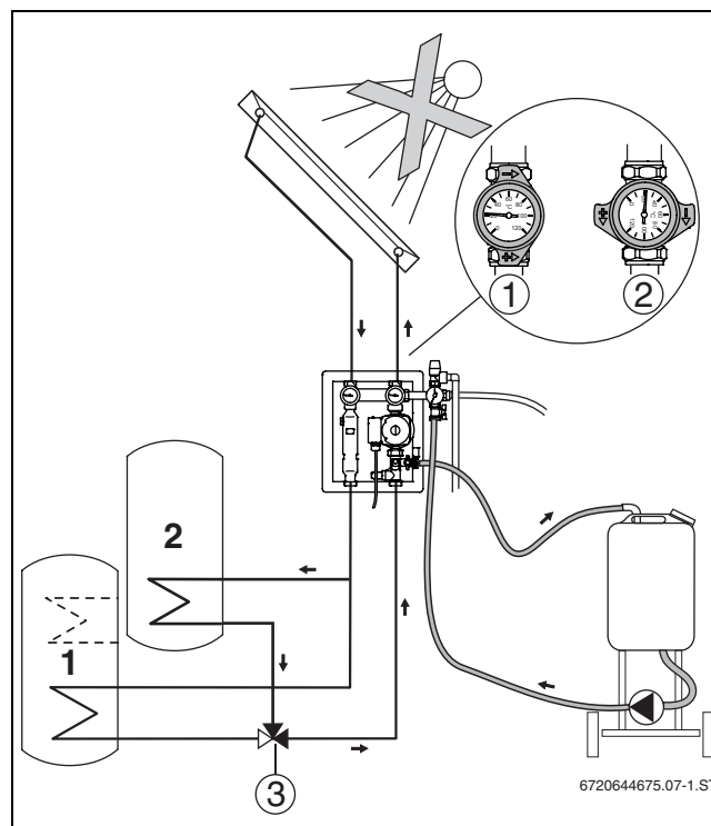
Fig. 7 de: Spülen bei Anlagen mit zwei Verbrauchern und Umschaltventil - hier: Spülen von Speicher 2 en: Flushing systems with two heat consumers and diverter valve - shown here: flushing cylinder 2
