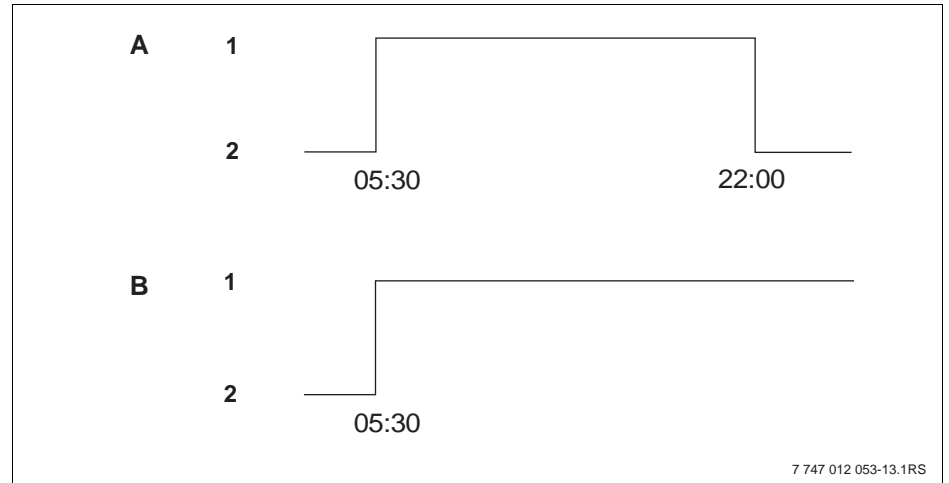
Bild 17 Schaltpunkt löschen
