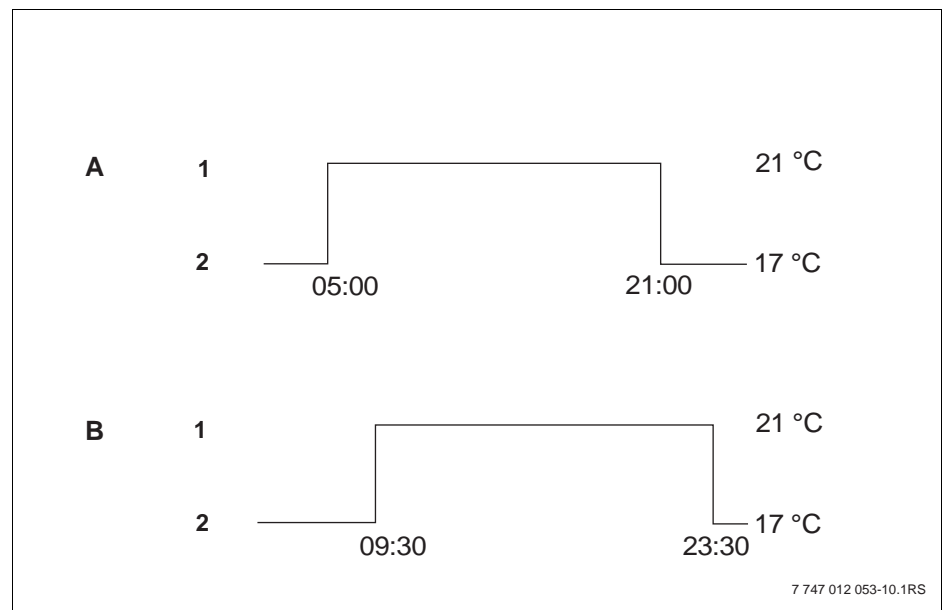
Bild 20 Neues Heizprogramm
