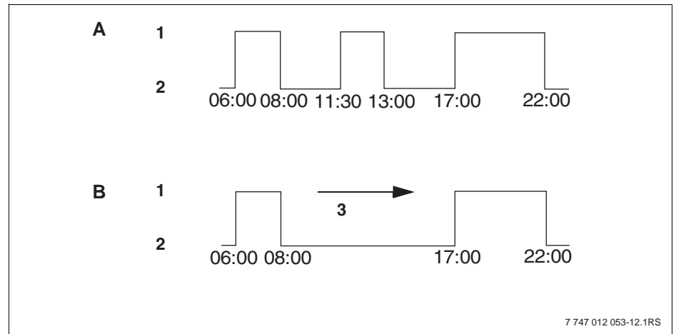
Bild 18 Heizphase löschen
