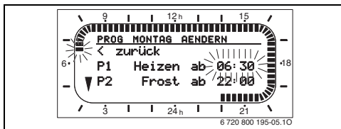
Bild 9 Schaltzeit einstellen
