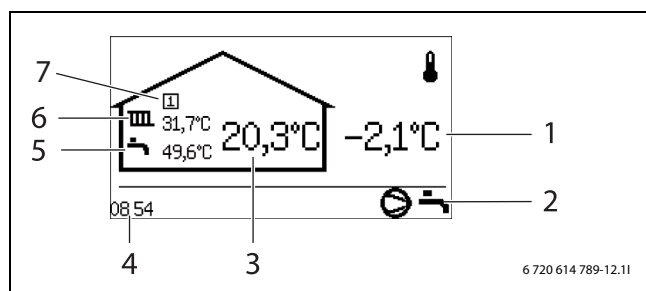
Bild 4 Standardanzeige
