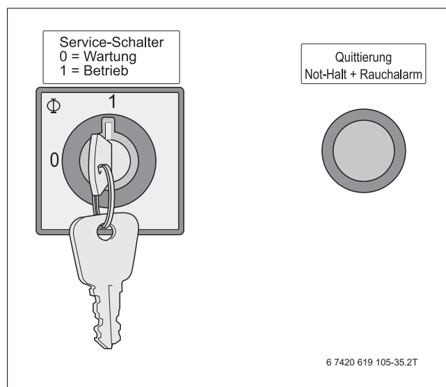
Bild 7 Serviceschalter in Stellung 1
