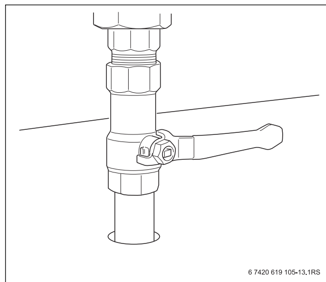
Bild 51 Gashahn geschlossen
