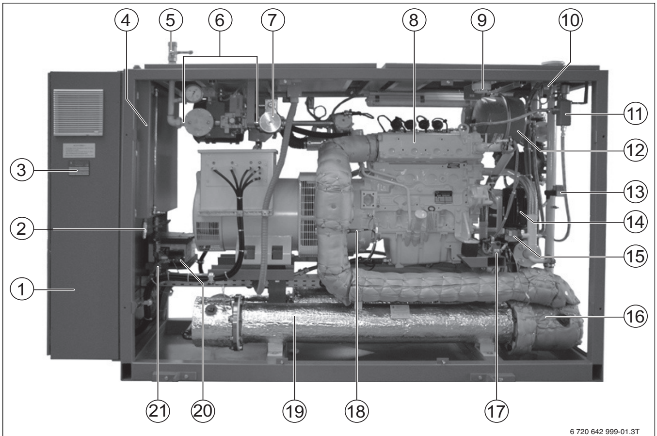
Bild 2 50 NA – Anlagenkomponenten Vorderansicht
