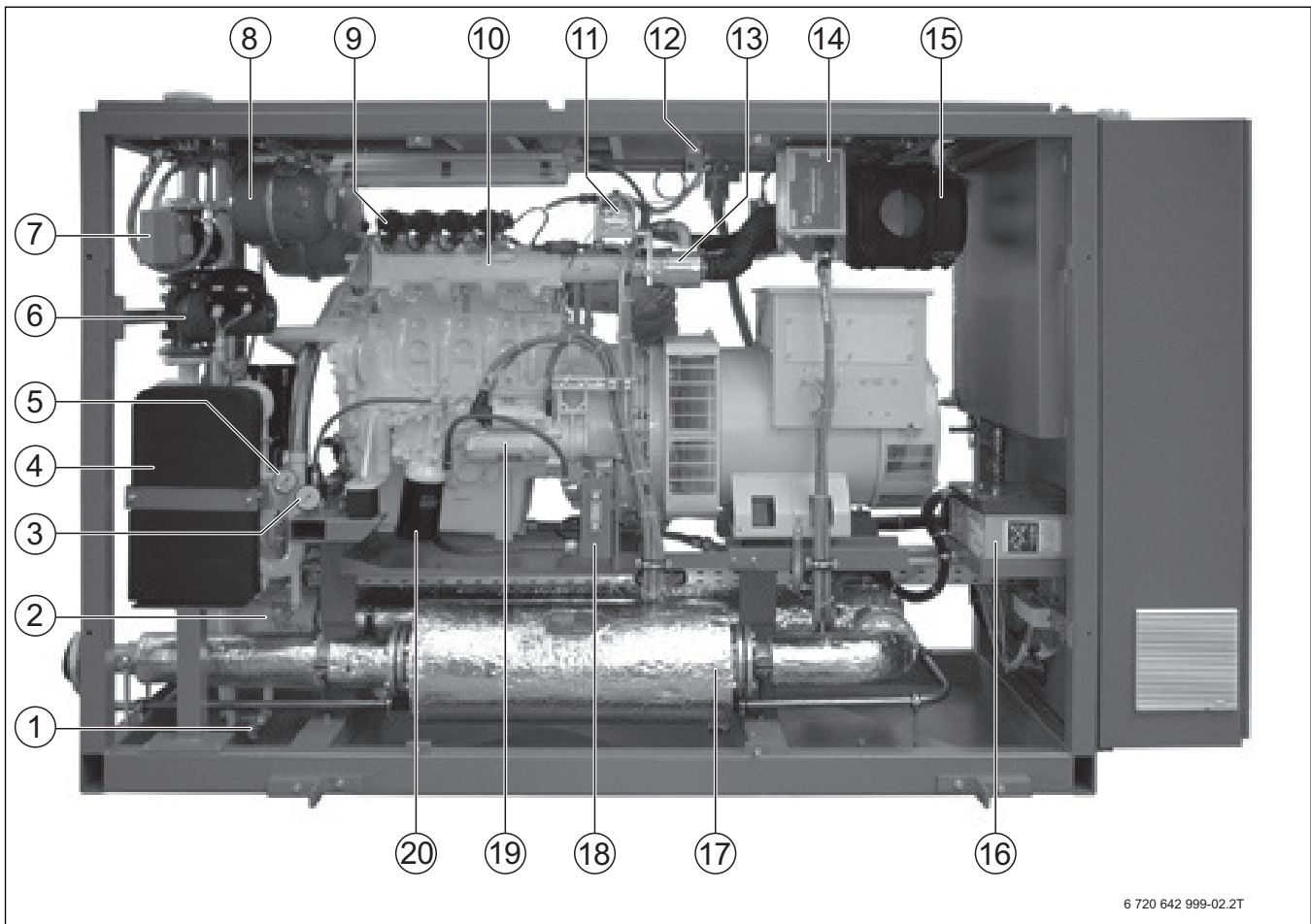
Bild 3 50 NA – Anlagenkomponenten Rückansicht
