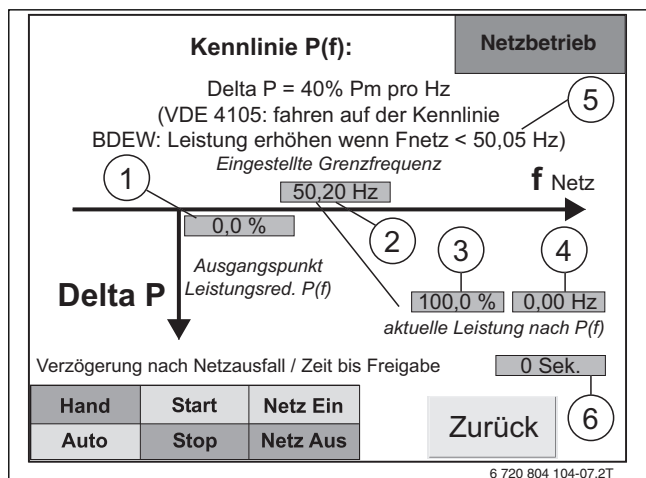
Bild 40 Beispiel "Leistungsreduzierung Fahren auf der Kennlinie P(f)"
