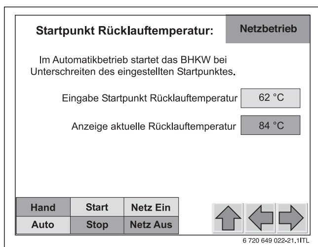
Bild 33 Einstellbild „Startpunkt Rücklauftemperatur“
