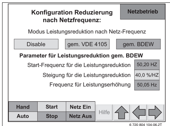
Bild 39 "Konfiguration Reduzierung nach Netzfrequenz" – gem. BDEW
