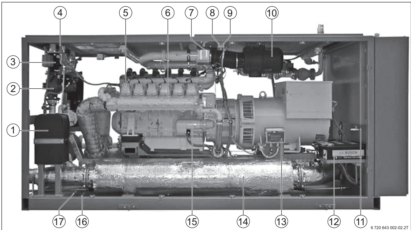
Bild 3 240 NA – Anlagenkomponenten Rückansicht
