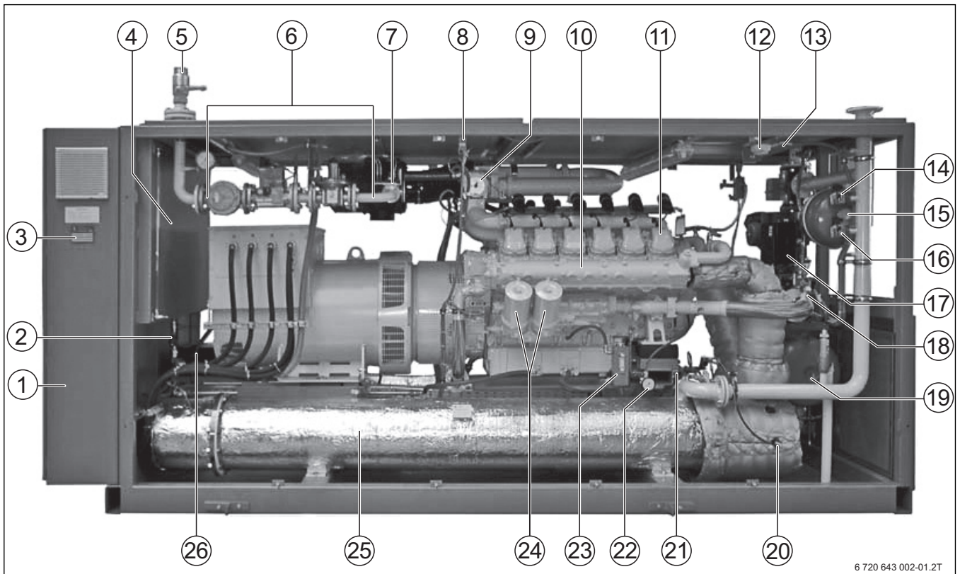
Bild 2 240 NA – Anlagenkomponenten Vorderansicht
