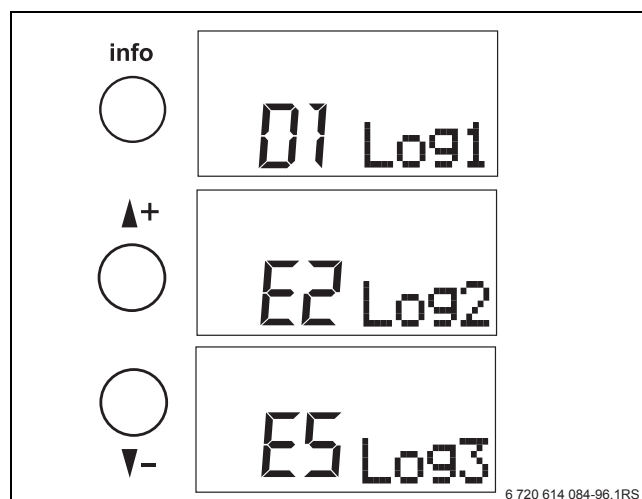
Bild 3 Störungshistorie
