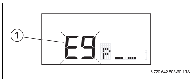
Bild 11 Display- und Störungs-Code
