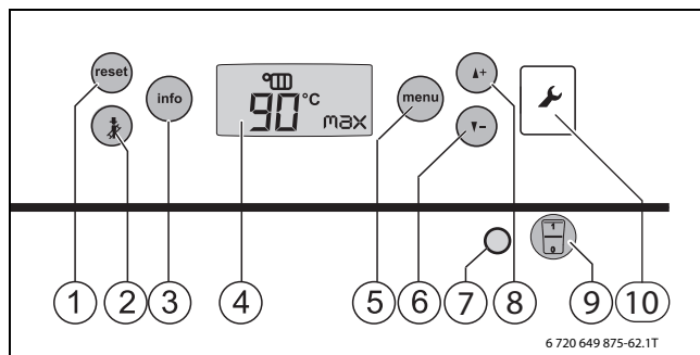
Bild 2 Bedienelemente
