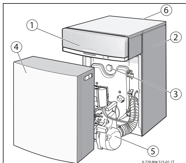
Bild 1 Hauptbestandteile des Kessels
