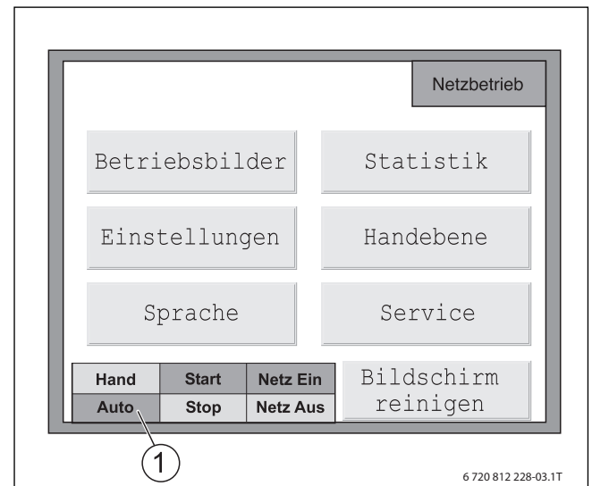
Bild 10 Einstellen Automatikbetrieb
