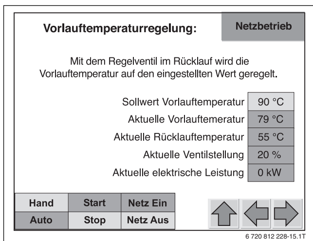
Bild 26 Einstellbild „Vorlauftemperaturregelung“
