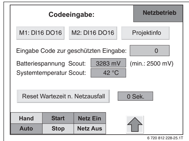
Bild 40 Service „Codeeingabe“
