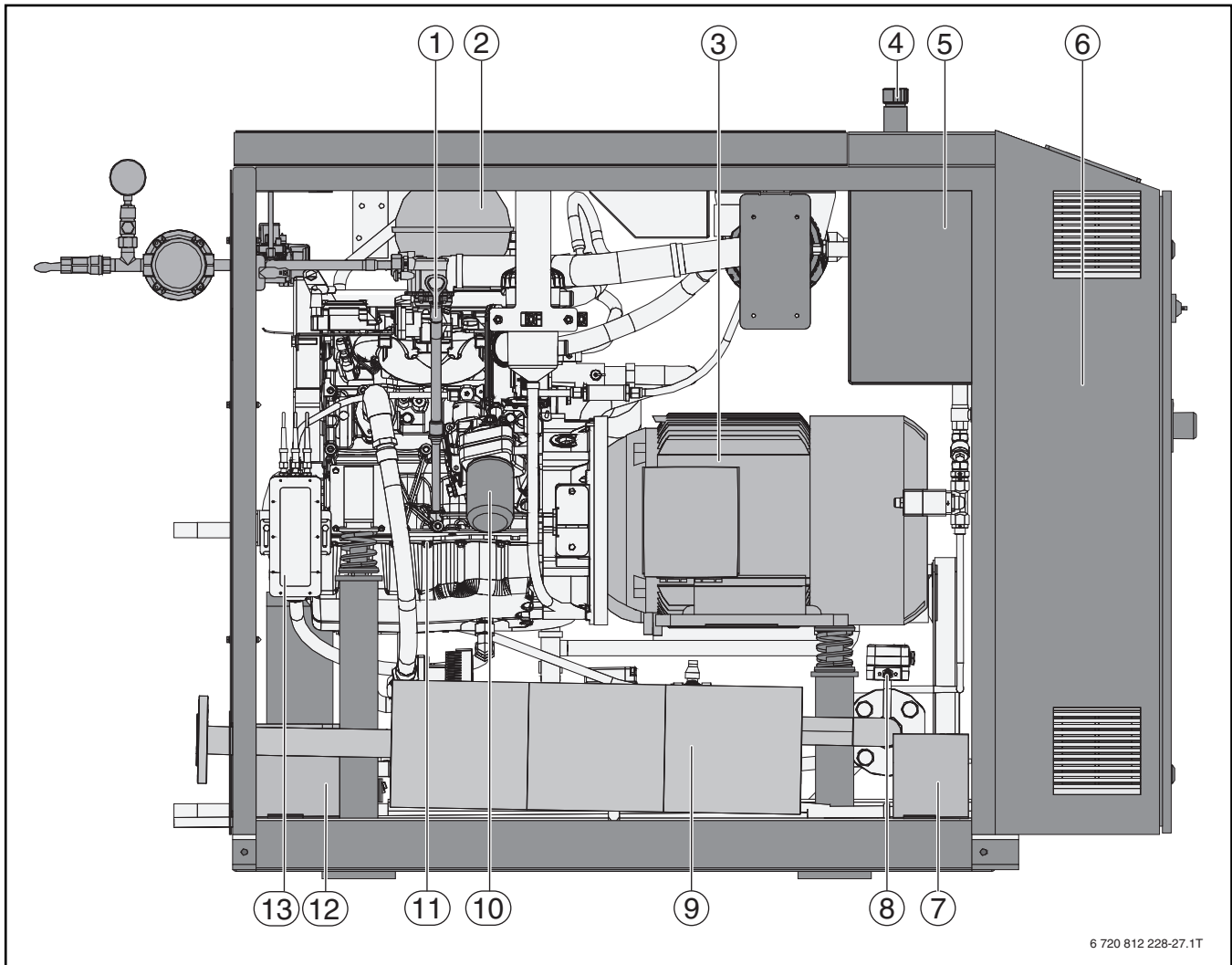
Bild 4 BHKW – Seitenansicht
