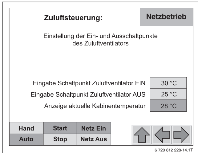
Bild 25 Einstellbild „Zuluftsteuerung“
