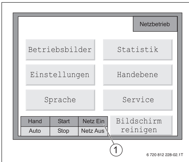
Bild 9 Generatorleistungsschalter zuschalten
