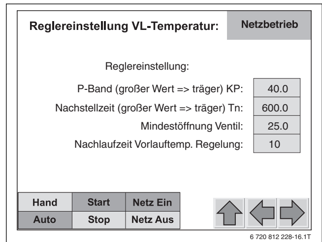
Bild 28 Einstellbild „Reglereinstellung VL-Temperatur“
