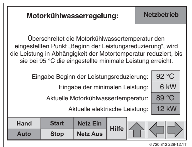
Bild 23 Einstellbild „Motorkühlwasserregelung“
