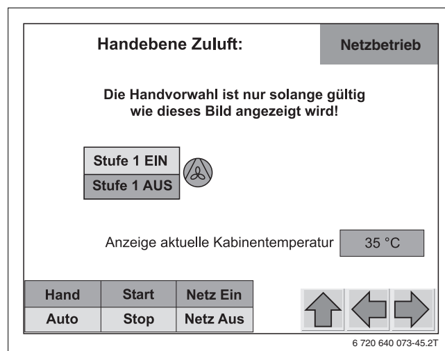
Bild 37 Handebene „Zuluft“
