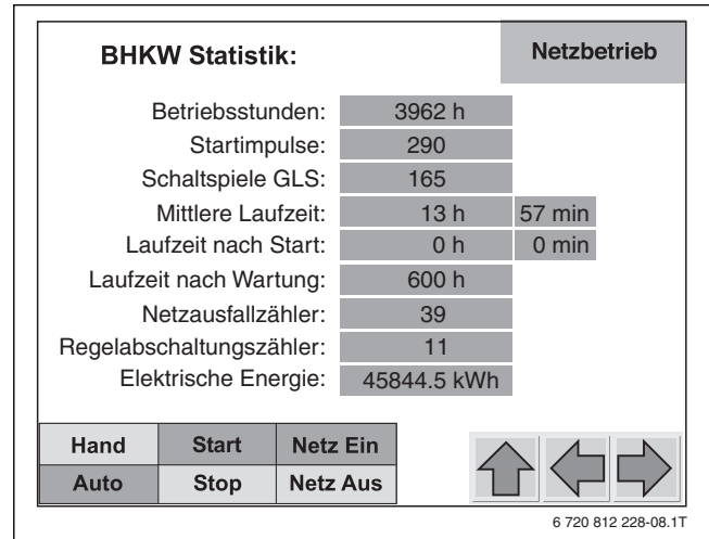
Bild 16 „BHKW Statistik“
