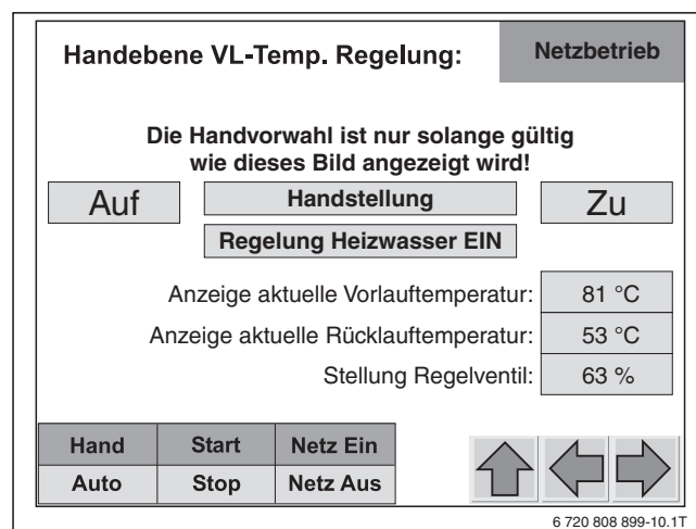
Bild 38 Handebene „Vorlauftemperaturregelung“
