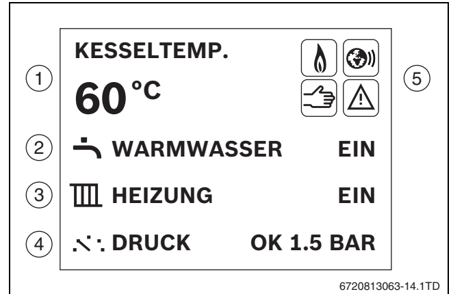
Bild 7 Standardanzeige
