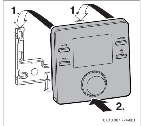
Bild 5 Bedieneinheit einhängen
