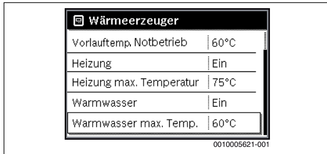
Bild 10 Maximale Warmwassertemperatur
