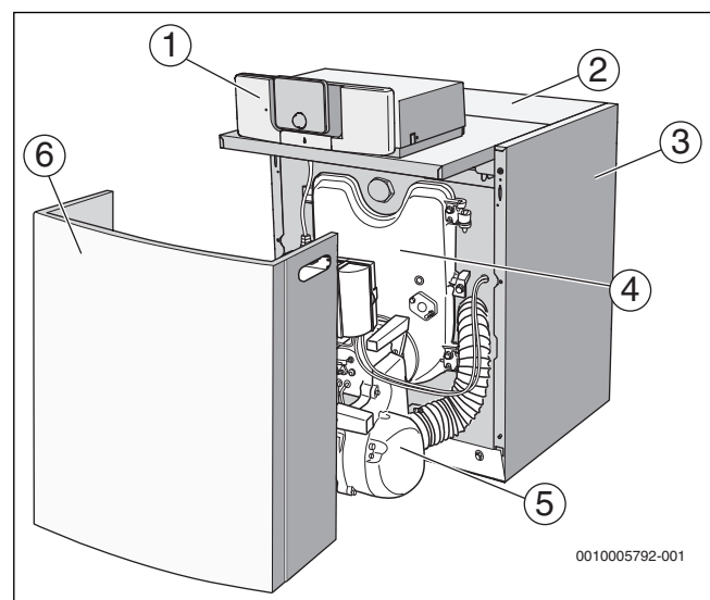
Bild 1 SuprapurCompact-O KUBC 18-1...49-1
