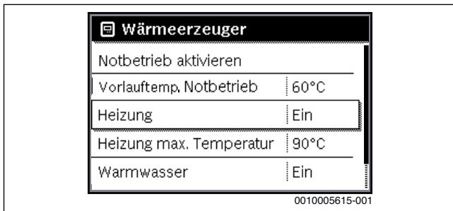
Bild 6 Heizung einschalten
