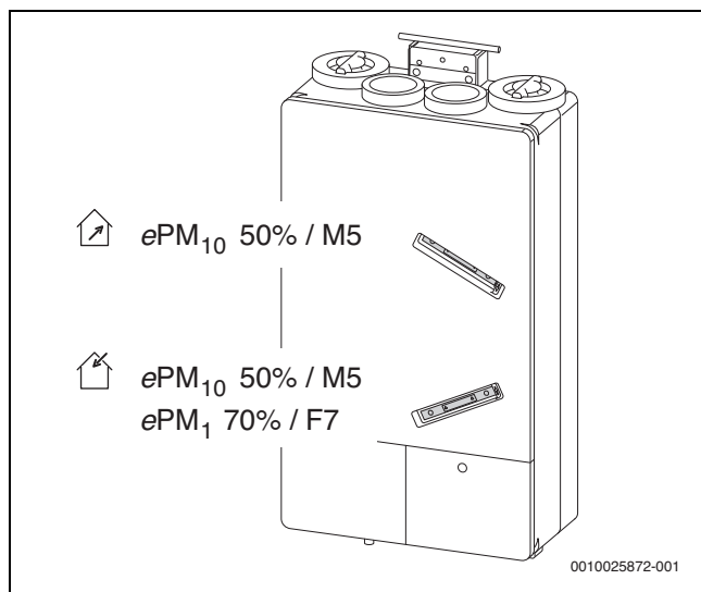
Bild 8 Filterposition
