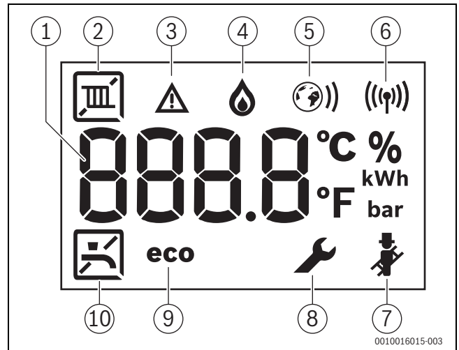
Bild 2 Displayanzeigen
