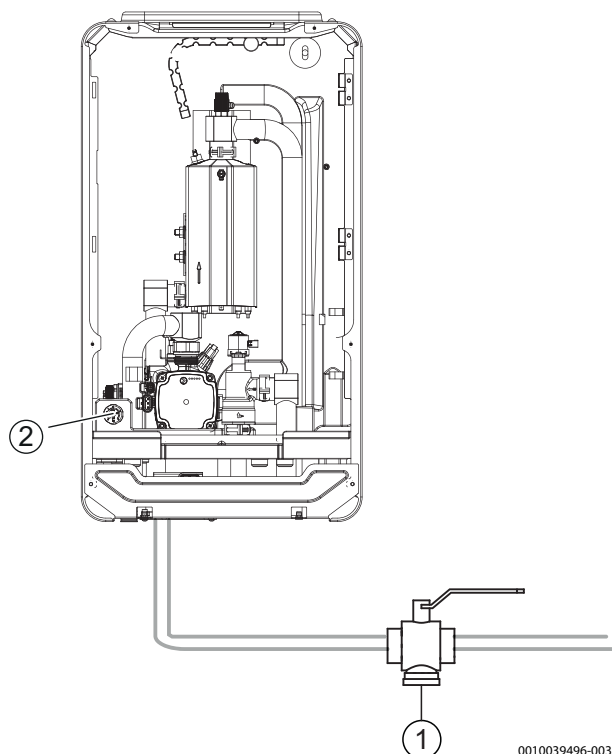
Bild 13 Inneneinheit Compress 5800/6800i 12 E
