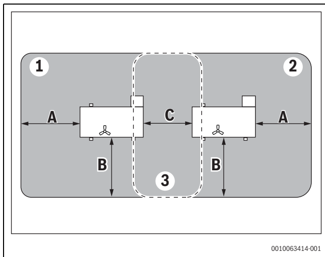
Bild 5 Überschneidung der Sicherheitsbereiche in einem Kaskadensystem
