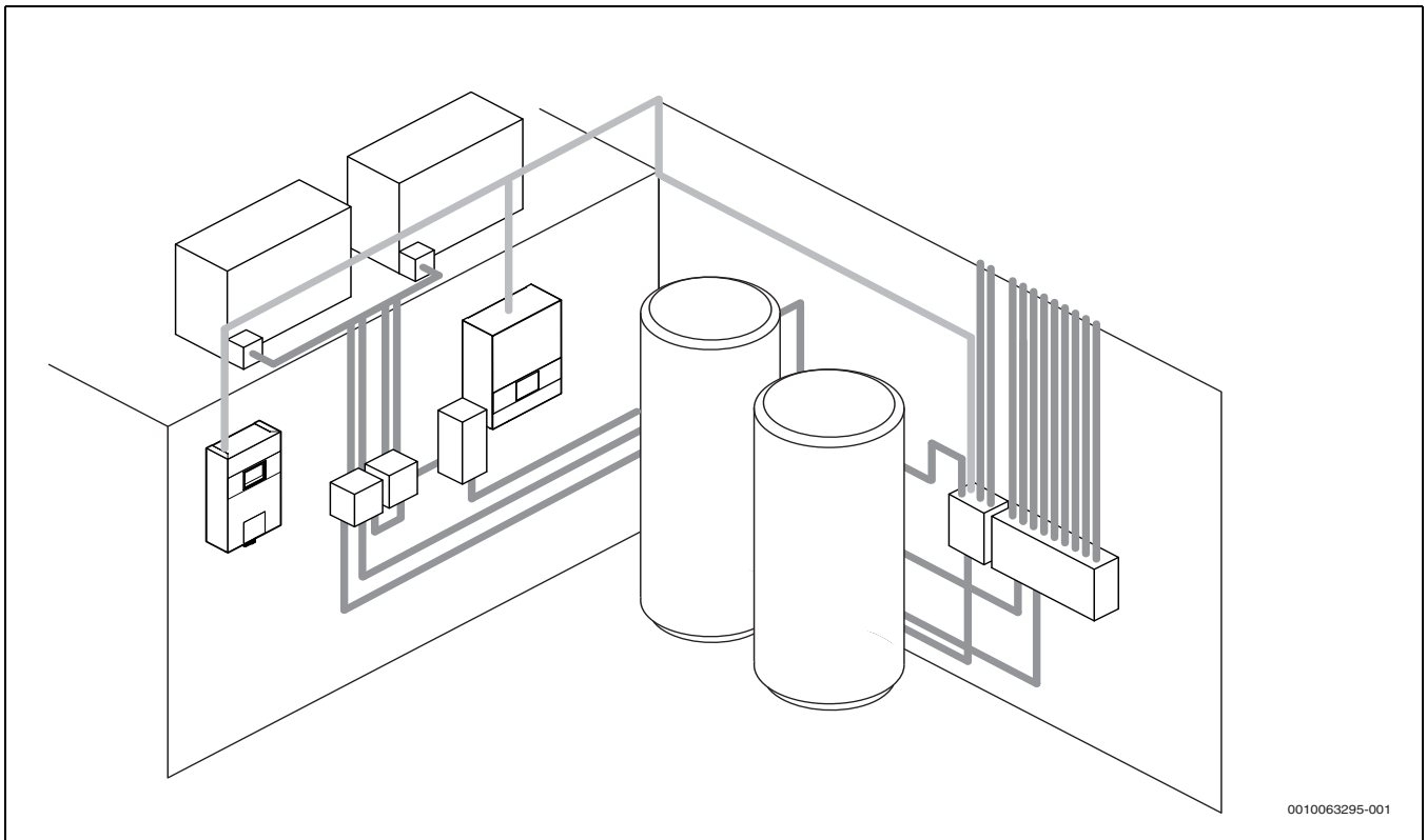
Bild 8 Außeneinheit, Wärmepumpenregler mit Zusatzheizung und externem Warmwasserspeicher
