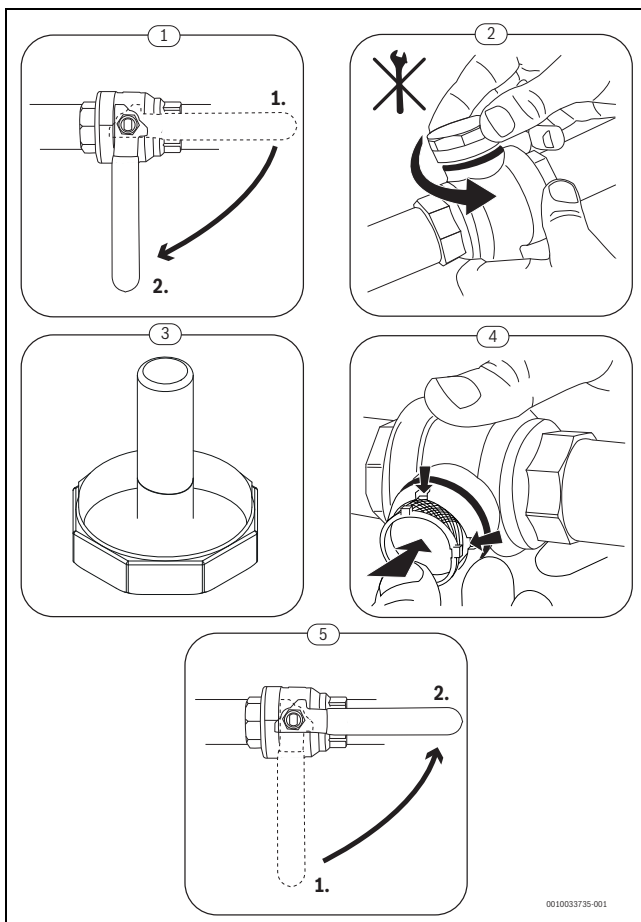
Bild 13 Reinigen des Partikelfilters
