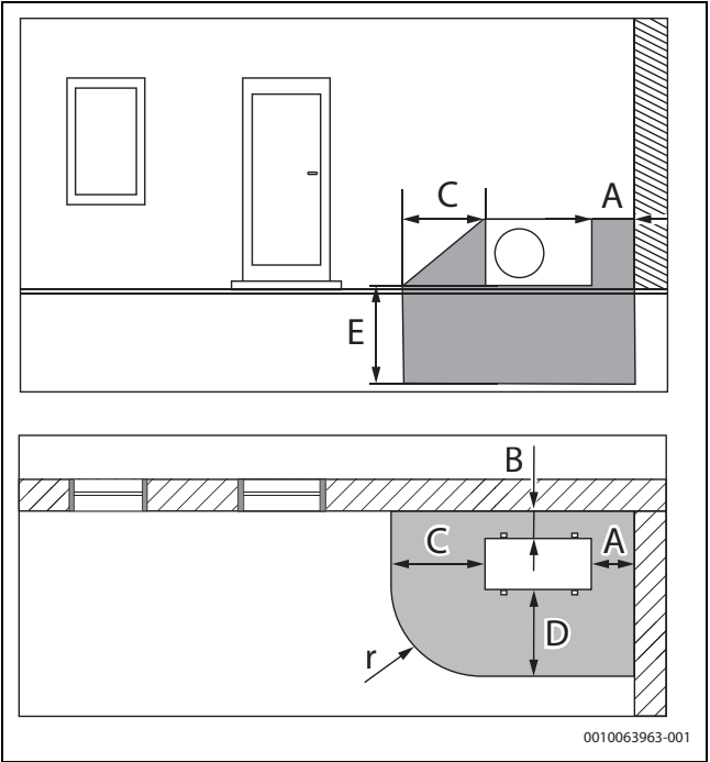
Bild 4 Sicherheitsbereich bei Carport-Montage der Wärmepumpe
