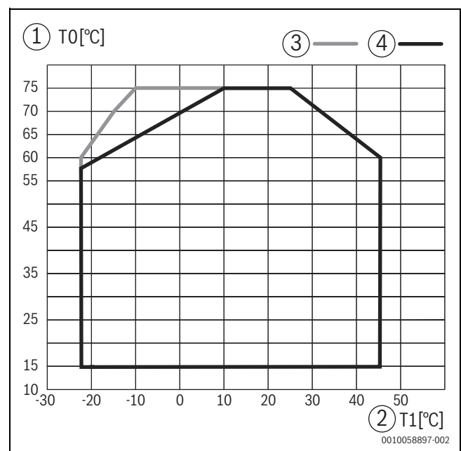
Bild 6 Wärmepumpe im Heizbetrieb ohne Zusatzheizung
