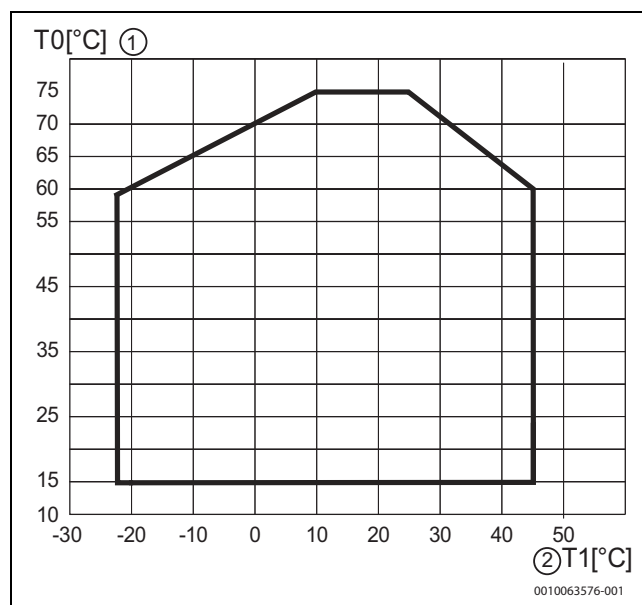
Bild 5 Wärmepumpe im Heizbetrieb ohne elektrischen Zuheizer
