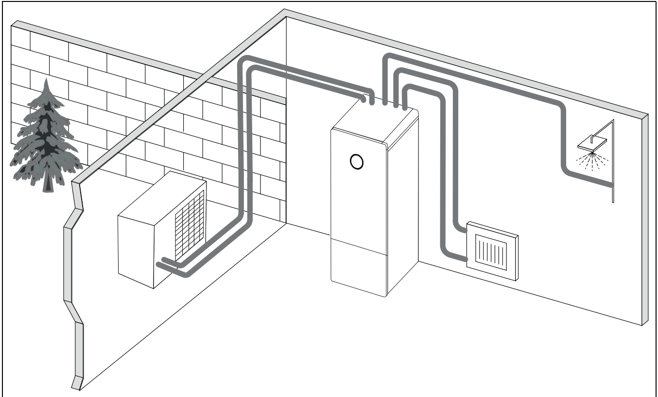
Bild 8 Wärmepumpe AW O, Inneneinheit Compress AWMMBi/D mit integriertem Warmwasserspeicher und elektrischem Zuheizer
