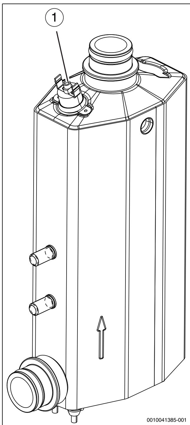
Bild 15 Überhitzungsschutz zurücksetzen
