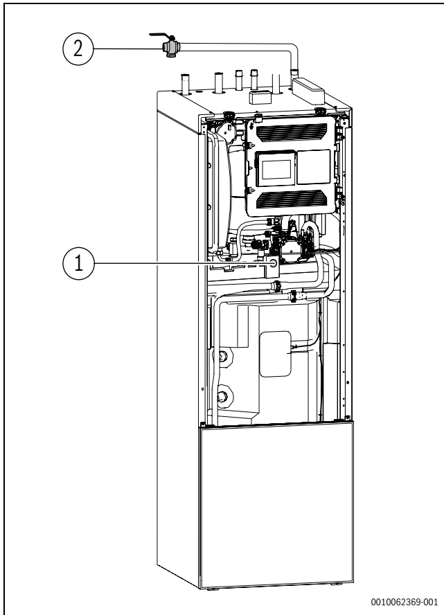
Bild 16 Compress AWMMBiD
