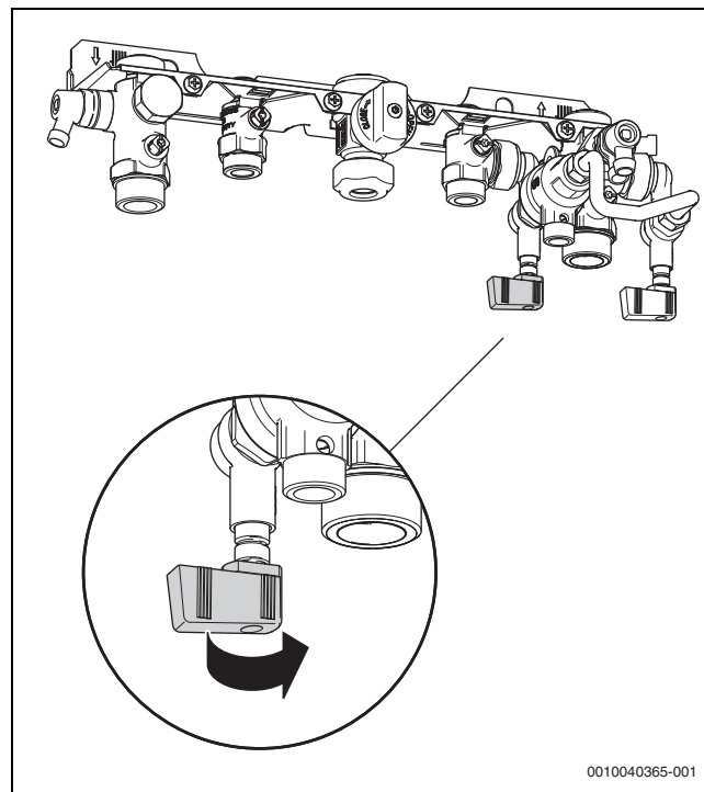
Bild 7 Fülleinrichtung öffnen
