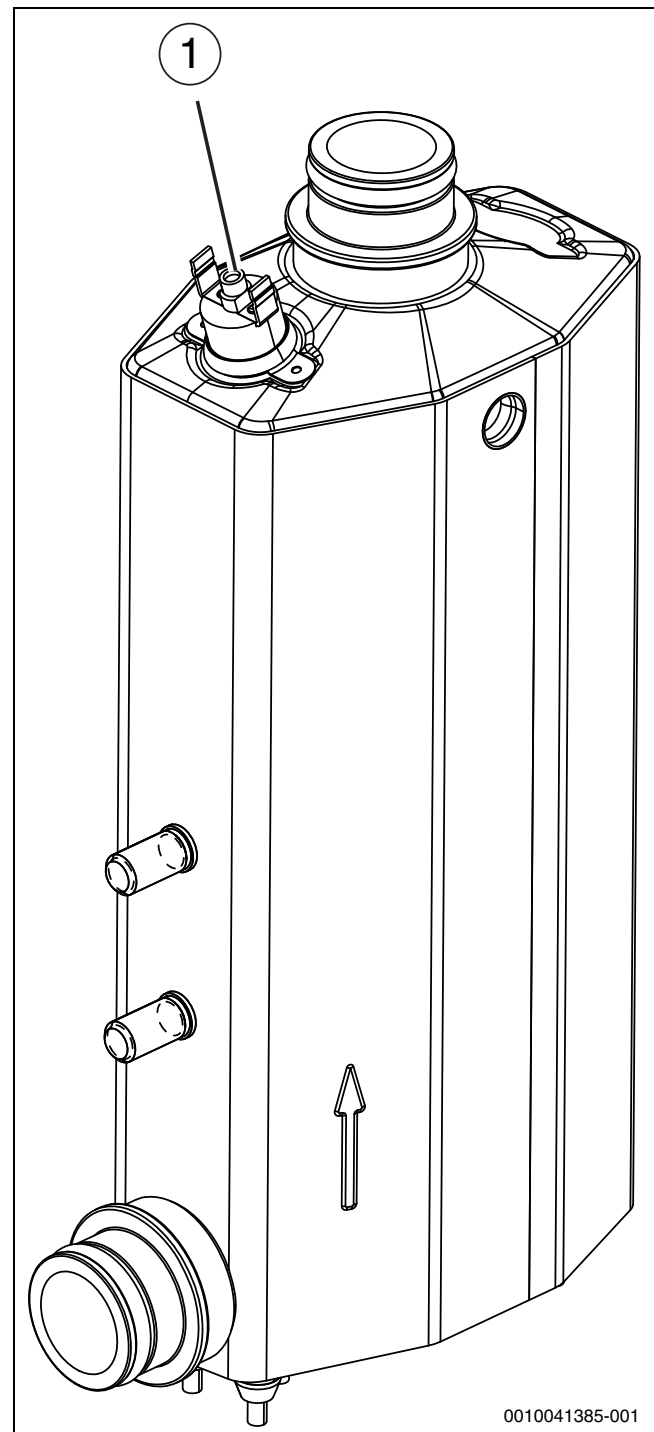
Bild 13 Überhitzungsschutz zurücksetzen
