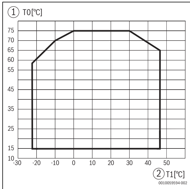
Bild 4 Wärmepumpe im Heizbetrieb ohne Zuheizung
