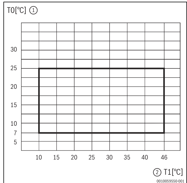
Bild 5 Wärmepumpe im Kühlbetrieb
