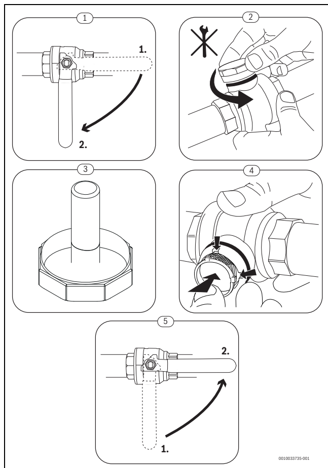
Bild 15 Reinigen des Partikelfilters
