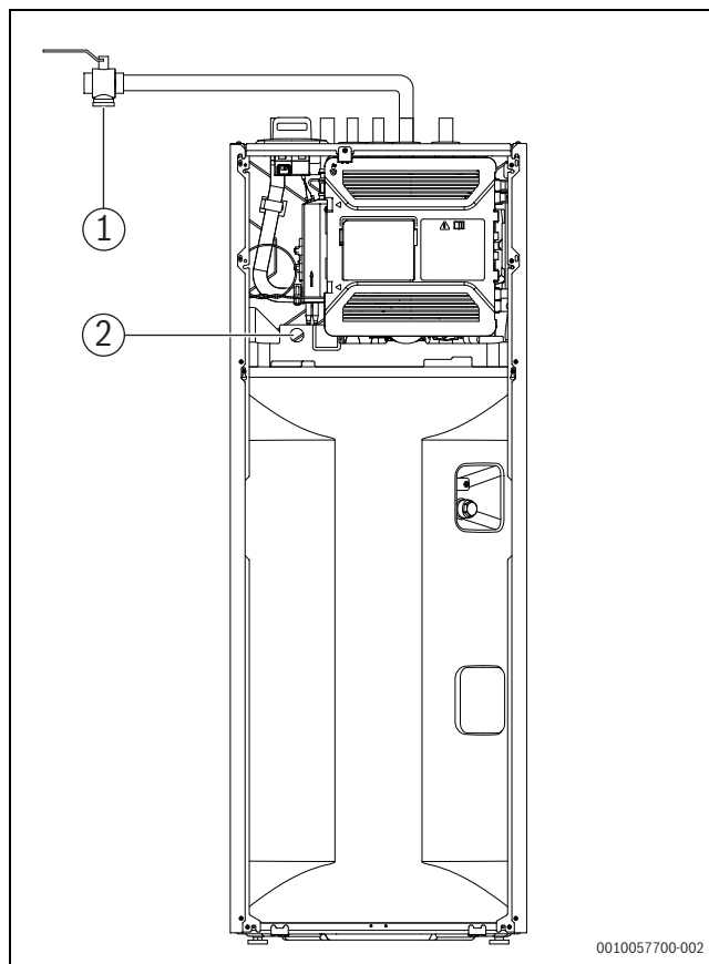
Bild 14 AWMi / AWMHi
