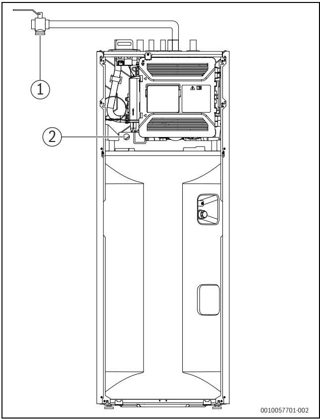
Bild 15 AWMi / AWMHi
