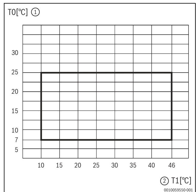
Bild 6 Wärmepumpe im Kühlbetrieb
