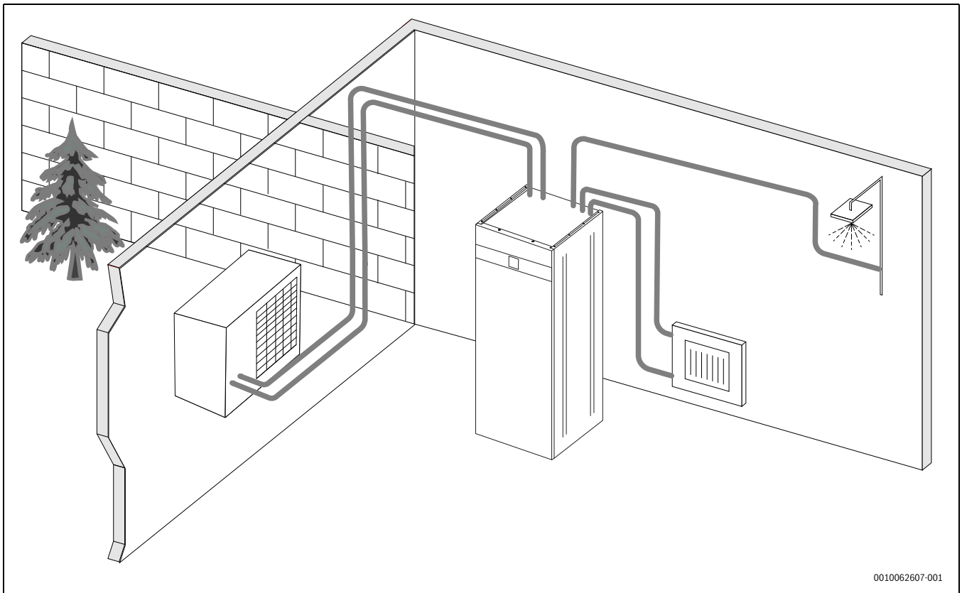
Bild 8 Außeneinheit, Inneneinheit mit Zuheizer und Warmwasserspeicher CS3800iAW O-S / CS3800iAW O-T
