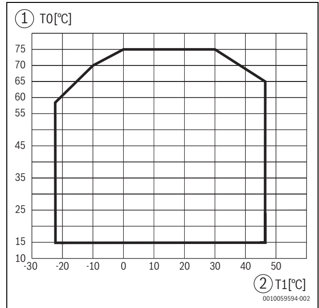
Bild 5 Wärmepumpe im Heizbetrieb ohne Zuheizung
