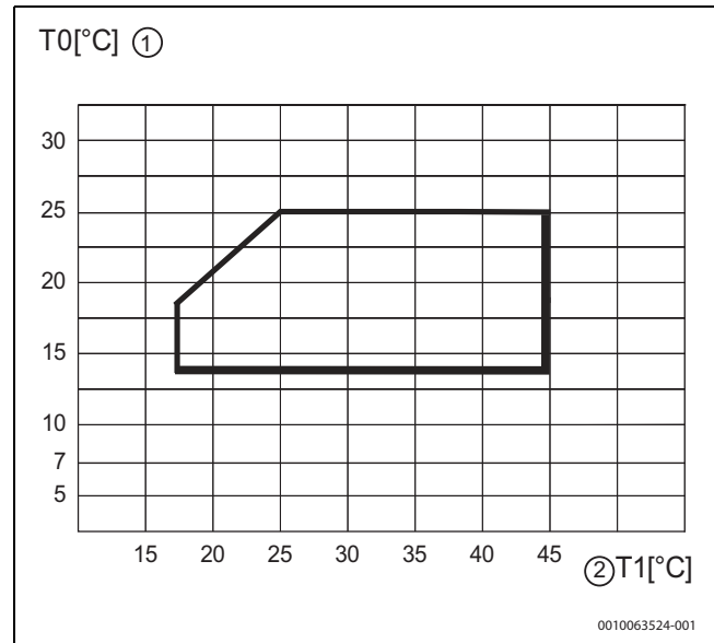
Bild 8 Wärmepumpe im Kühlbetrieb CS5801iAW O-S / CS5801iAW O-T / CS8800iAW O-T
