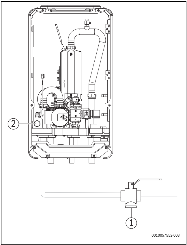
Bild 17 Inneneinheit
