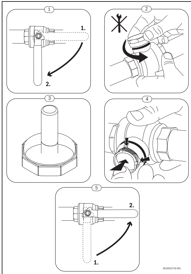
Bild 18 Reinigen des Partikelfilters
