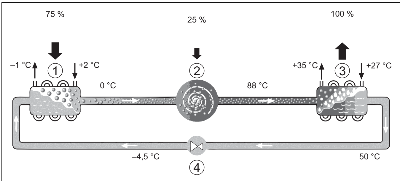
Bild 9 Funktionsprinzip des Kältemittelkreises in der Wärmepumpe
