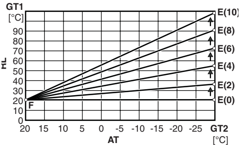
Bild 16 Anheben des Endpunkts der Heizkurve
