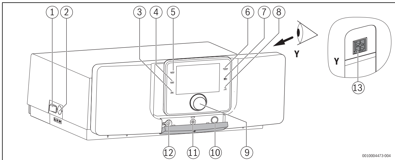
Bild 3 Regelgerät MX25 mit Bedieneinheit – Bedienelemente
