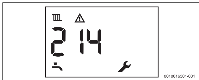
Bild 6 Beispiel eines Störungsdisplayes
