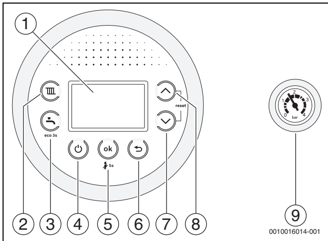
Bild 1 Bedienfeldübersicht
